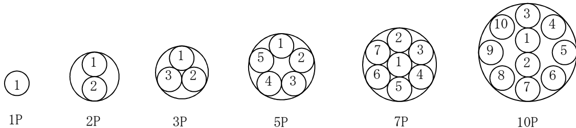
配 列 図
