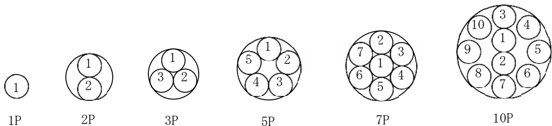
配 列 図
