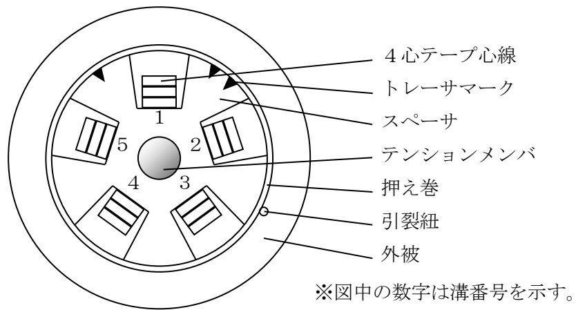
図3. ケーブル構造図 (28心~60心)
