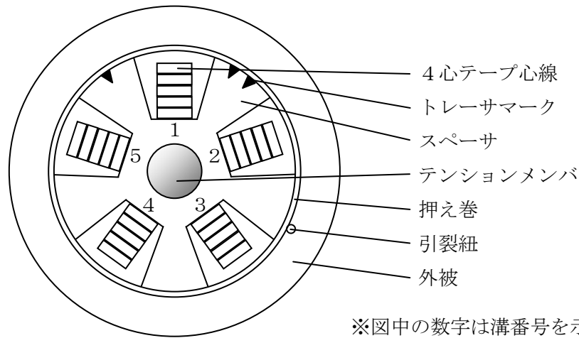
図5. ケーブル構造図 (64心~100心)
