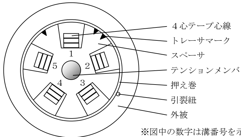
図4. ケーブル構造図 (44～60心)
