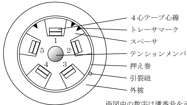
図3. ケーブル構造図 (28～40心)
