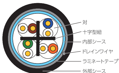
構造図
