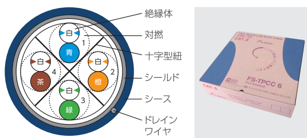
構造図
