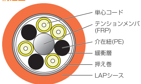
構造図
