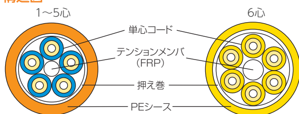
構造図
