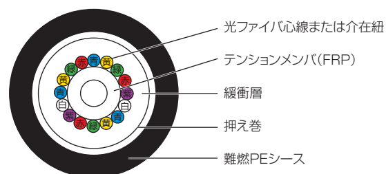
構造図
