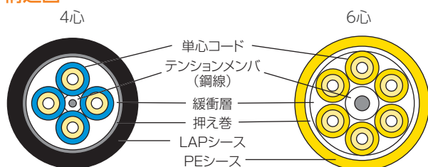
構造図
