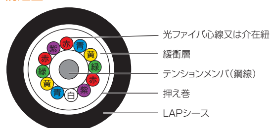
構造図
