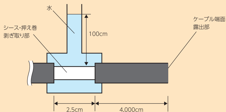
図2. 試験方法
