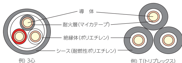
構造表
